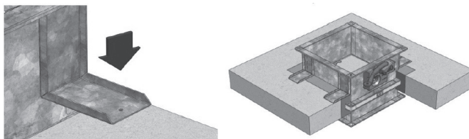
obrázek č. 5 – instalace požární clapky do pevného stropu
