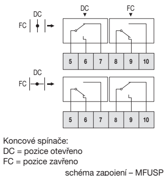
schéma zapojení – MFUSP
