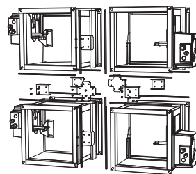
obrázek č. 7 – instalace skupiny požárních clapek v tzv. baterii
