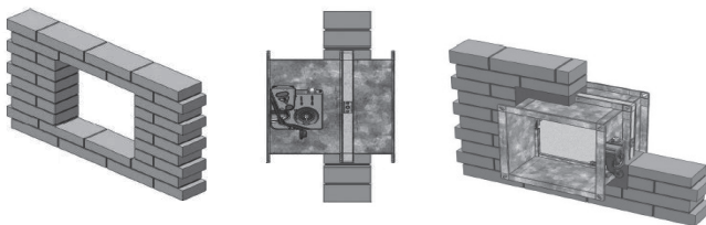
obrázek č. 3 – instalace požární clapky v pevné konstrukci
