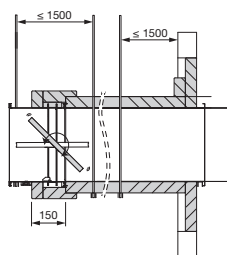
obrázek č. 6 – instalace požární clapky mimo požární dělicí konstrukci
