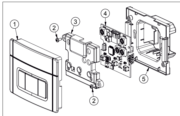
Obrázek 18. Rozložené schéma ovladače NASHIRA S
