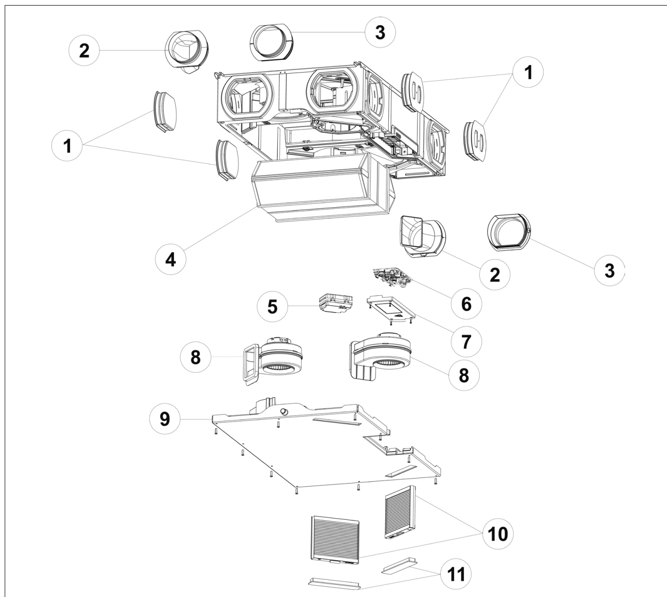
Obrázek 19. Rozložené schéma NASHIRA S
