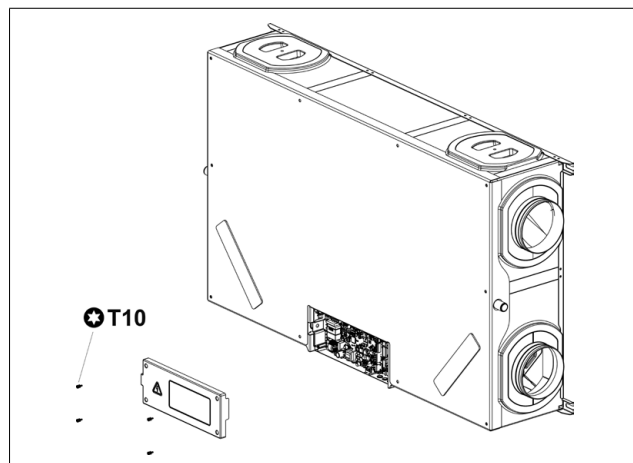
Obrázek 17. Vyjmutí PCB
