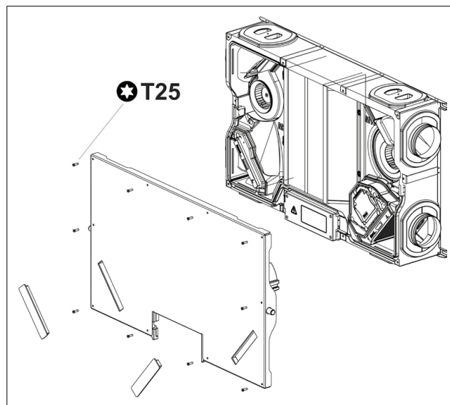
Obrázek 5. Demontáž předního krytu
