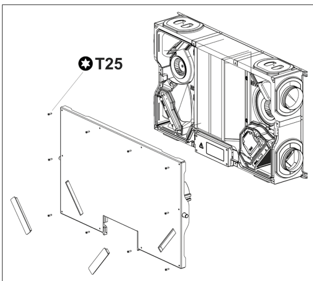
Obrázek 8. Demontáž předního krytu
