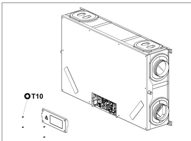
Obrázek 16. Odstranění krytu elektroniky
