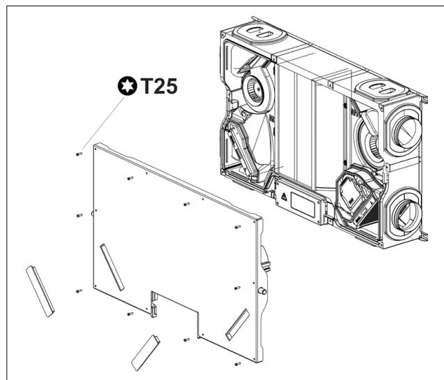
Obrázek 11. Demontáž předního krytu
