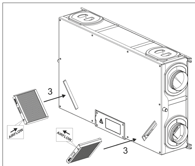
Obrázek 3. Vložte nové filtry
