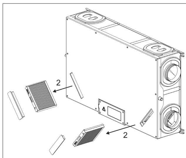
Obrázek 2. Vyjmutí filtrů
