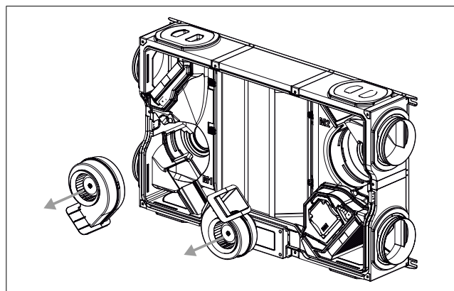
Obrázek 12. Odstranění ventilátorů
