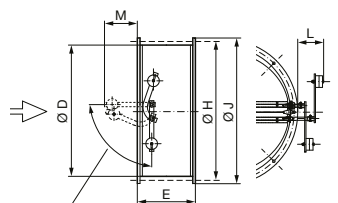
TSK 630–1250 (pouze vodorovně)
