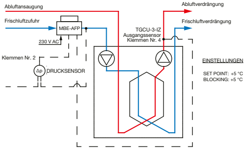
Technologische Schema des Anschlusses der Elektroheizung im Vorheizmodus (Frostschutz des Geräts) mit einem externen NTC-Tempersensoren ( T_s \geq 5 \text{ °C} Einstellwert SET POINT, T_b \geq 5 \text{ °C} Einstellwert BLOCKING)
