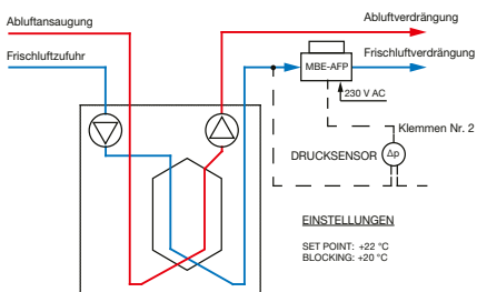
technologisches Schema für den Anschluss des Elektroheizers im Zuluft-Nacherwärmungsmodus ( T_s \geq 22 \text{ °C} Einstellwert SET POINT, T_b \geq 20 \text{ °C} Einstellwert BLOCKING)
