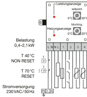
Technologische Schema des Anschlusses der Elektroheizung im Vorheizmodus (Frostschutz des Geräts) mit einem externen NTC-Tempersensoren ( T_s \geq 5 \text{ °C} Einstellwert SET POINT, T_b \geq 5 \text{ °C} Einstellwert BLOCKING)
