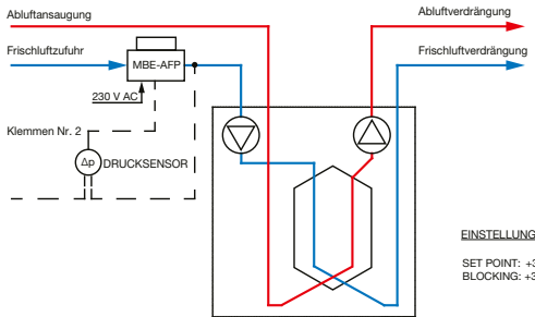
Technologische Schema des Anschlusses der Elektroheizung im Vorheizmodus (Frostschutz des Geräts) ohne Verwendung eines externen NTC-Tempersensoren ( T_s \geq 3 \text{ °C} Einstellwert SET POINT, T_b \geq 3 \text{ °C} Einstellwert BLOCKING)
