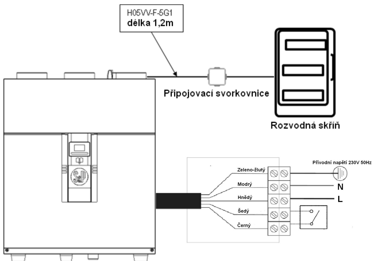
Schéma 1 – zapojení jednotky
