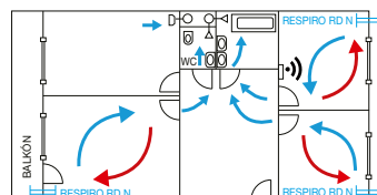
schematický náčrt větrání místností v bytu s použitím větrací jednotky s regenerací RESPIRO N RD
