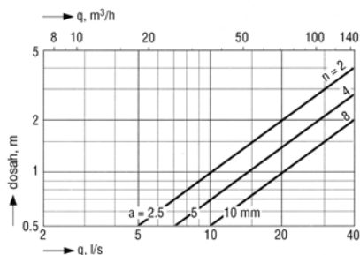
VST 80
