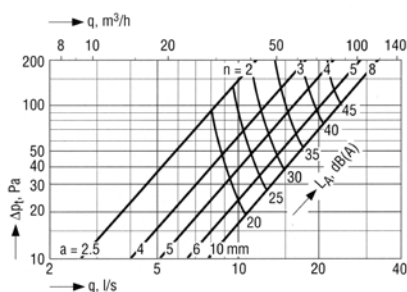
VST 100
