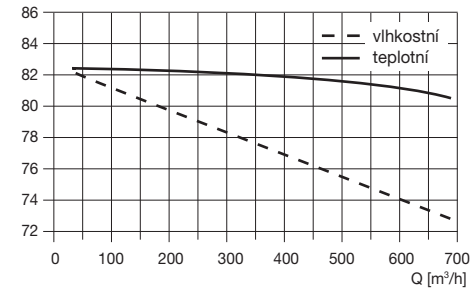
η [%] Graf účinnosti
