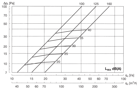
Diagram pro dimenzování ventilů
