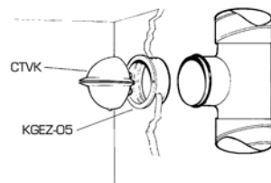
příklady montáže
