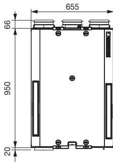
zadní pohled
