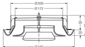
VEF 200
