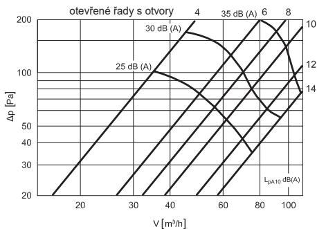
WDZA 125 – přívod
