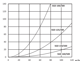
tlaková ztráta
