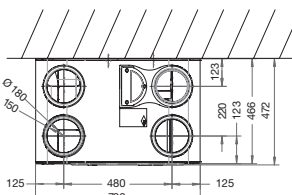
pohled shora – připojovací hrdla
