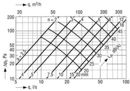
VST 160
