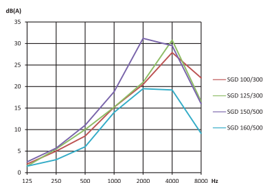
vložný útlum
