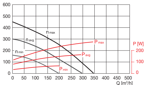
Pst [Pa] Rovento 320
