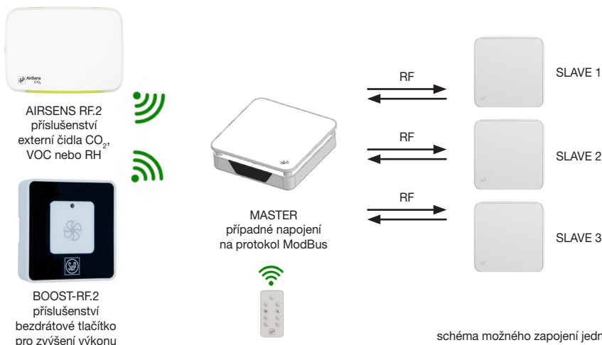
schéma možného zapojení jednotek NARAH 160 s dalším příslušenstvím v jedné sestavě
