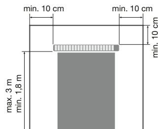
Montagehöhe und Wandabstand
