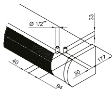
Detail des Wasseranschlusses für COR-NW Blenden
