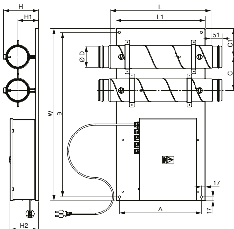
Ausführung "O"
