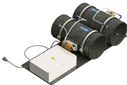
Ausführung "O"
