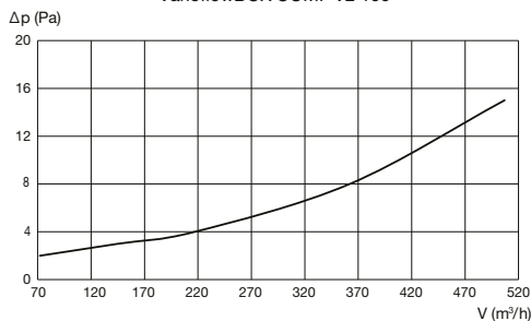
VarioflowBOX COMF V2 160
