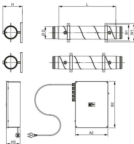
Ausführung "R"
