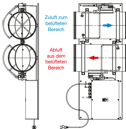
rechte Ausführung
