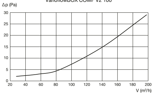
VarioflowBOX COMF V2 100
