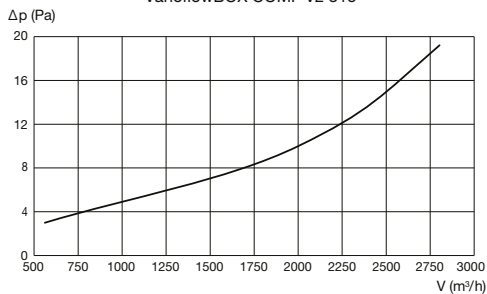
VarioflowBOX COMF V2 315
