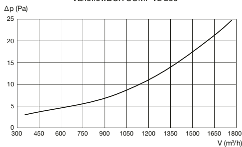
VarioflowBOX COMF V2 250
