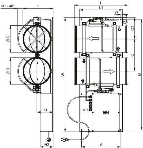
Ausführung "O"
