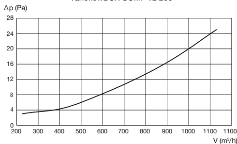
VarioflowBOX COMF V2 200
