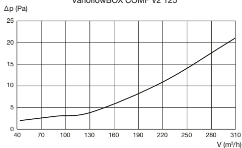
VarioflowBOX COMF V2 125
