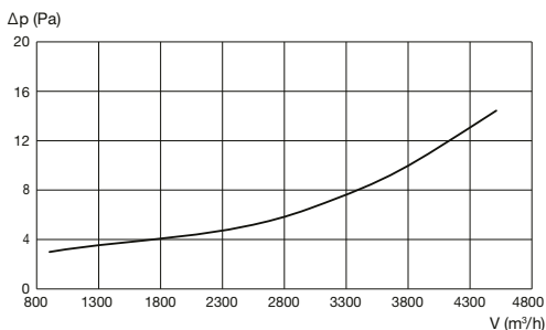
VarioflowBOX COMF V2 400
