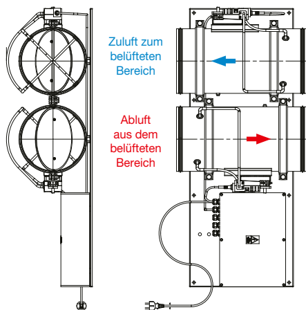
linke Ausführung
