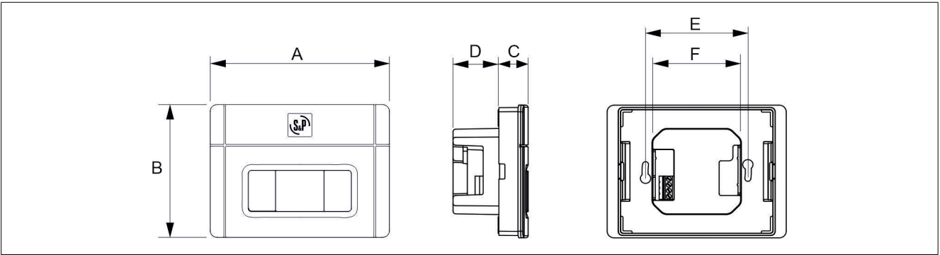
Obrázek 4. Schéma rozměrů ovladače
