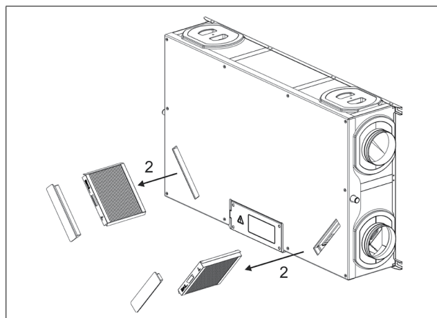
Obrázek 2. Vymutí filtrů
