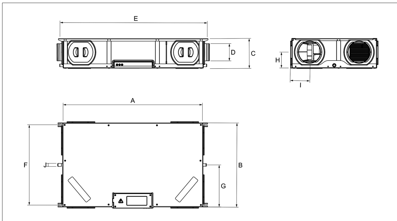
Obrázek 3. Schéma rozměrů NASHIRA S
