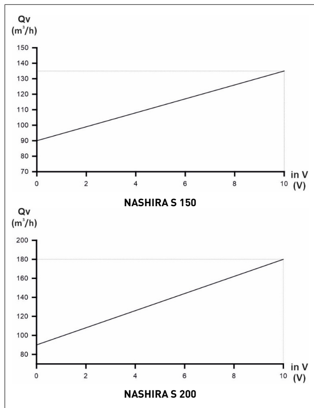
Obrázek 16. Proporční režim [V] NASHIRA S 150 a 200
