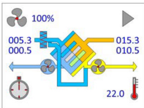
předehřev aktivní
