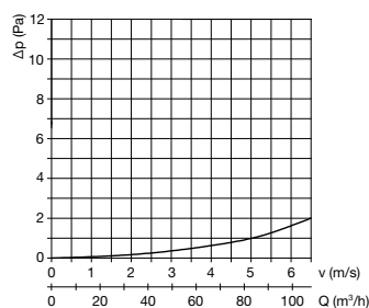
ED Flex® 90/77 PRO pro 1 m rovného potrubí
