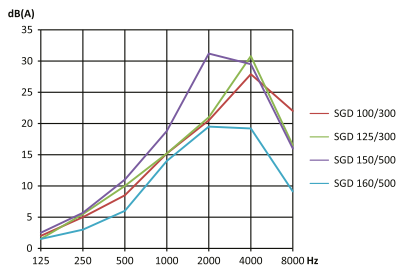
vložený útlum
