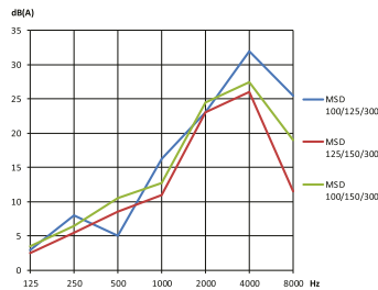
vložený útlum
