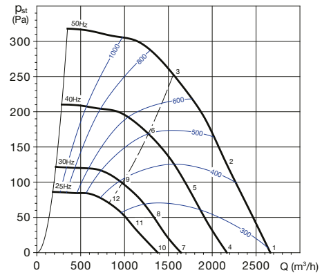
CTVT/4-250 N
