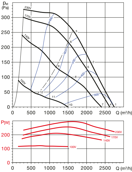
CTHB/4-250 N
