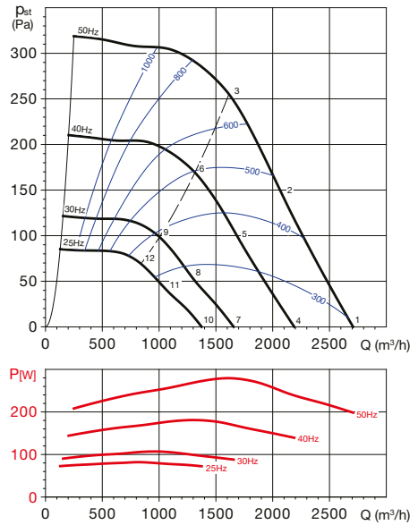
CTHT/4-250 N
