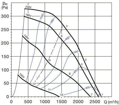
CTVB/4-250 N
