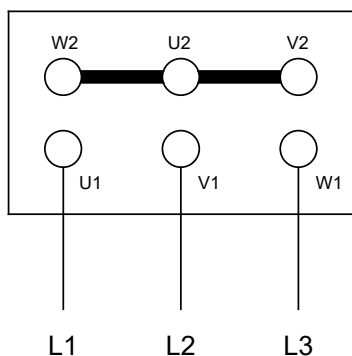
zapojení Y
