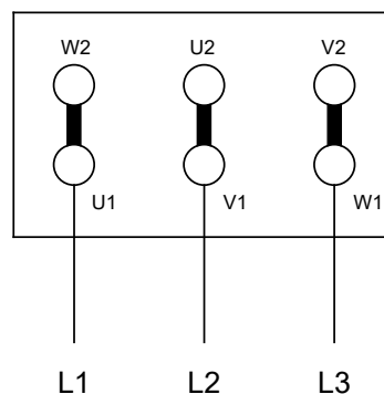
zapojení Δ
