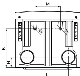
hrdlo pro výtlak čerstvého vzduchu (varianta A)
