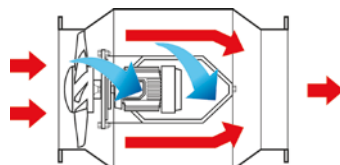
motor je uložen mimo proud vzduchu v kanále umístěném kolmo ve skříni ventilátoru, chlazen je ventilátorem, který je jeho konstrukční součástí
