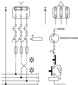
Schaltplan CMPT Y oder Δ Schaltung je nach Typenschild und geliefertem Motortyp
