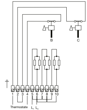
Schaltplan 2x 400V
