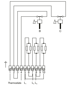
Schaltplan, 3x 400V
