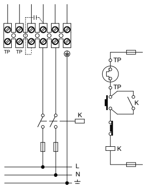
CVAB 250 připojení ventilátoru k síti
