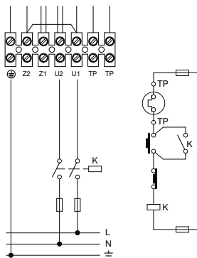
CVAB 315-450 připojení ventilátoru k síti
