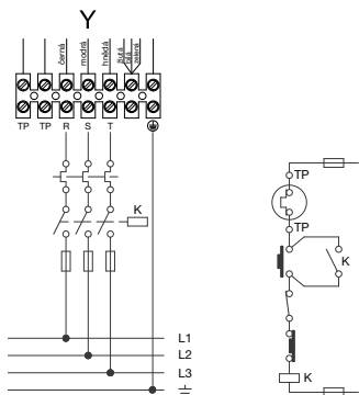
CVAT 250 připojení ventilátoru k síti
