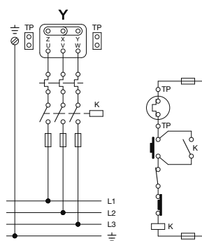
CVAT 710, 800 připojení ventilátoru k síti
