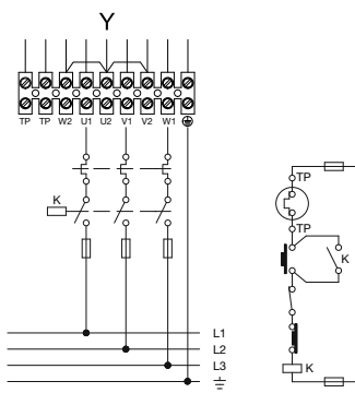
CVAT 315-630 připojení ventilátoru k síti
