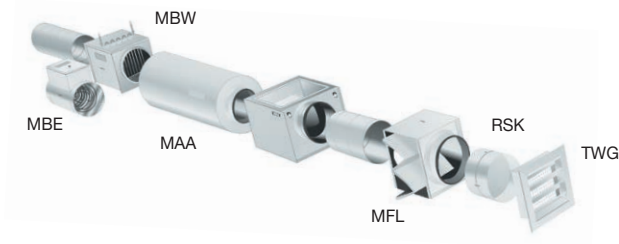
přívodní sestava
