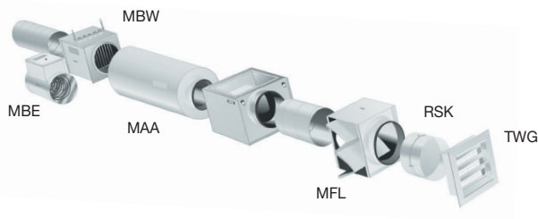
přívodní sestava
