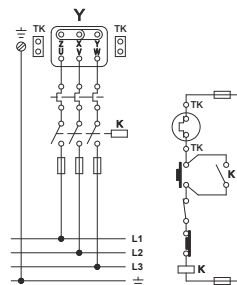
připojení ventilátoru k síti 3x400V
