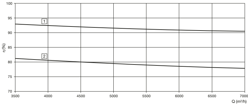
DUOVENT® COMPACT DV 6900 - Wirkungsgrad der Rückgewinnung
