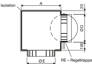
Anschlusskasten PDCI-G mit Außenisolierung (Dicke 6 mm)
