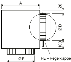
Anschlusskasten PDC-G
