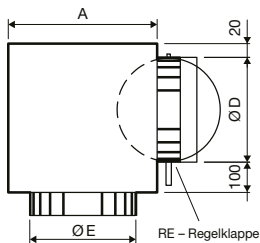
Anschlusskasten PDC
