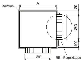
Anschlusskasten PDCI
