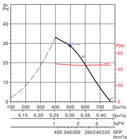
HXTR-TXTR/4-250
