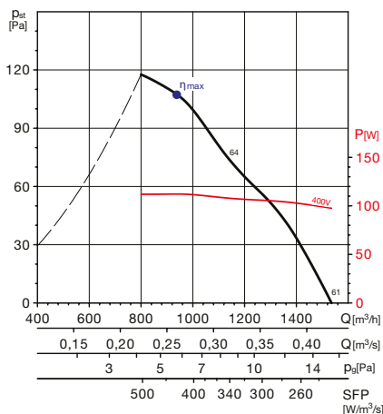
HXTR-TXTR/2-250
