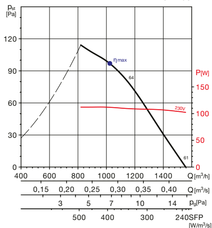
HXBR-TXBR/2-250
