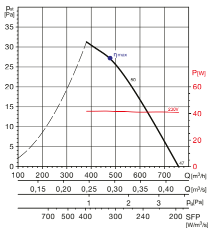
HXBR-TXBR/4-250
