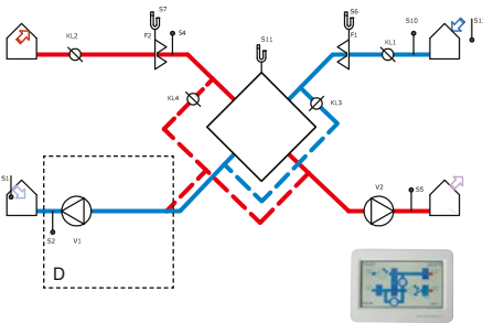
Plattenwärmetauscher
