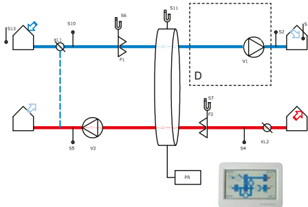
Rotationswärmetauscher
