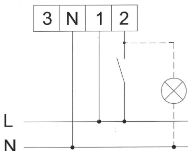
obr. 7 - schéma zapojení
