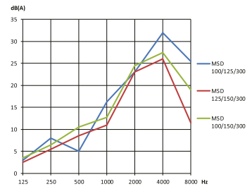
Einfügungsdämpfung
