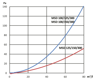
Druckverlust
