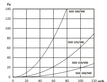
Druckverlust
