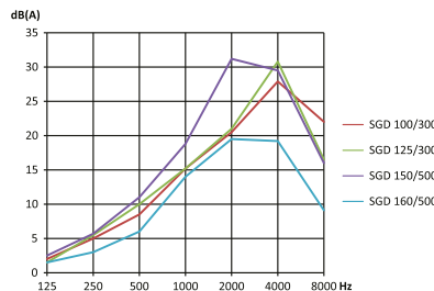
Einfügungsdämpfung
