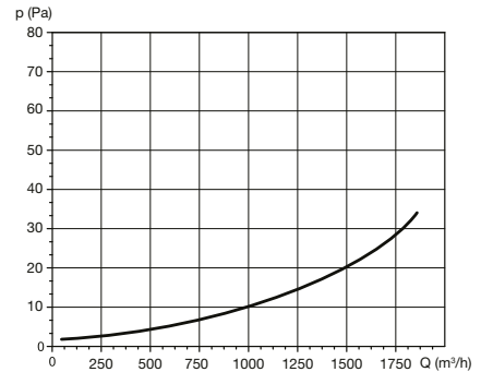
Druckverlustwerte des Dachsammlers VH 315 abhängig von der Luftströmung im Druckrohr (Richtwerte)
