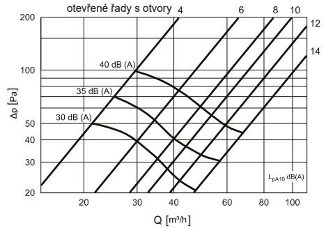
WDZA 125 – odvod
