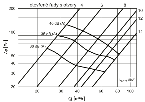
Diagramy tlakových ztrát bez osazených filtrů
