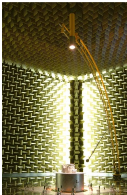
Akustická komora
