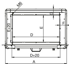
RME 2400; 3000; 4000; 6000 - poloha H1
