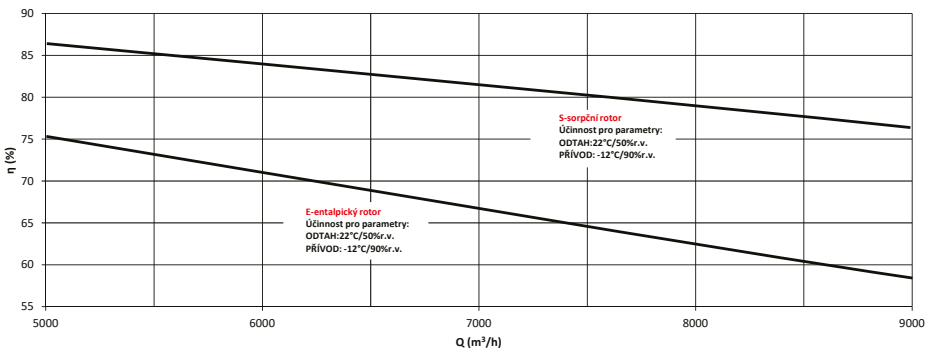
DUOVENT® MODULAR RV 8500 - VLHKOSTNÍ ÚČINNOST REGENERACE
