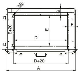
RMW 2400; 3000; 4000; 6000 - poloha H1
