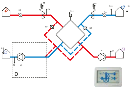
deskový výměník
