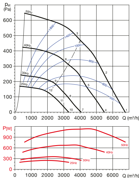
CTVT/4-400 N
