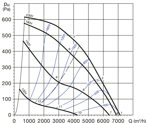
CTHB/4-400 N
