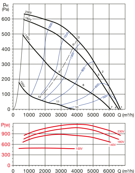
CTVB/4-400 N
