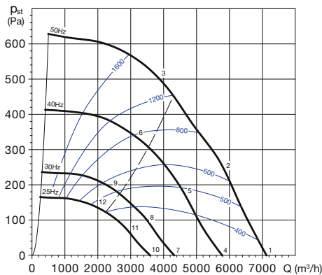
CTHT/4-400 N
