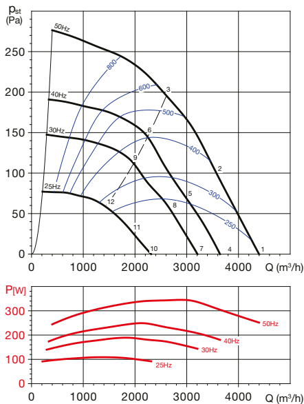
CTVT/6-400 N
