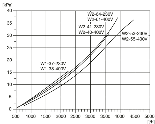
tlakové ztráty vodních výměníků
