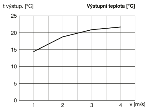
Závislost výstupní teploty vzduchu na rychlosti průtoku vzduchu
