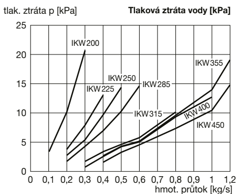
Tlaková ztráta vody [kPa]
