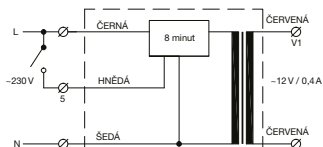
vnitřní zapojení CTE 12/708
