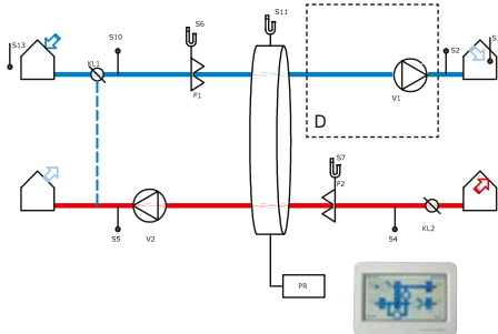
Rotationswärmetauscher
