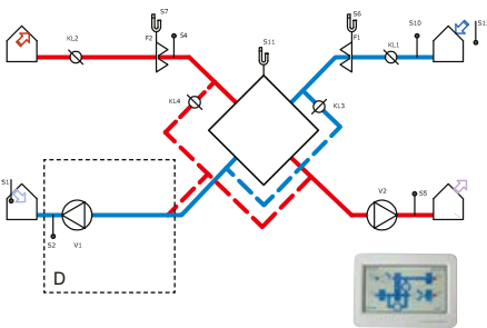
Plattenwärmetauscher
