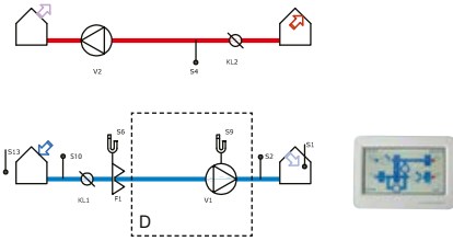
Zuluft- + Abluftgerät
